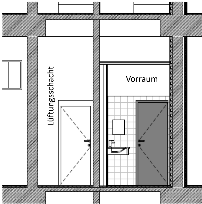
Schnitt Vorraum
