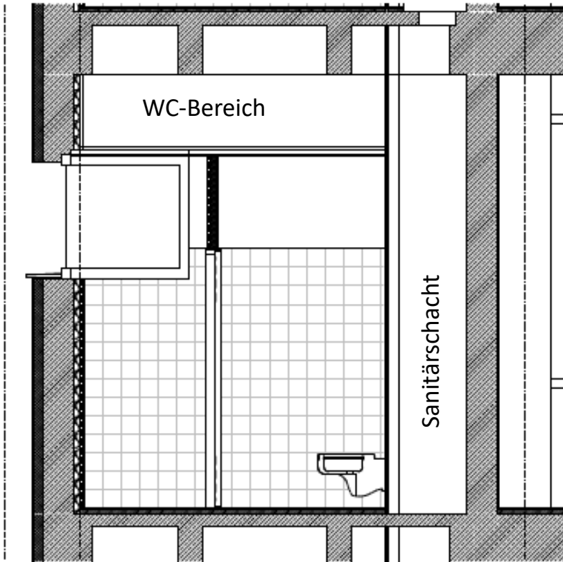
Schnitt WC-Bereich
