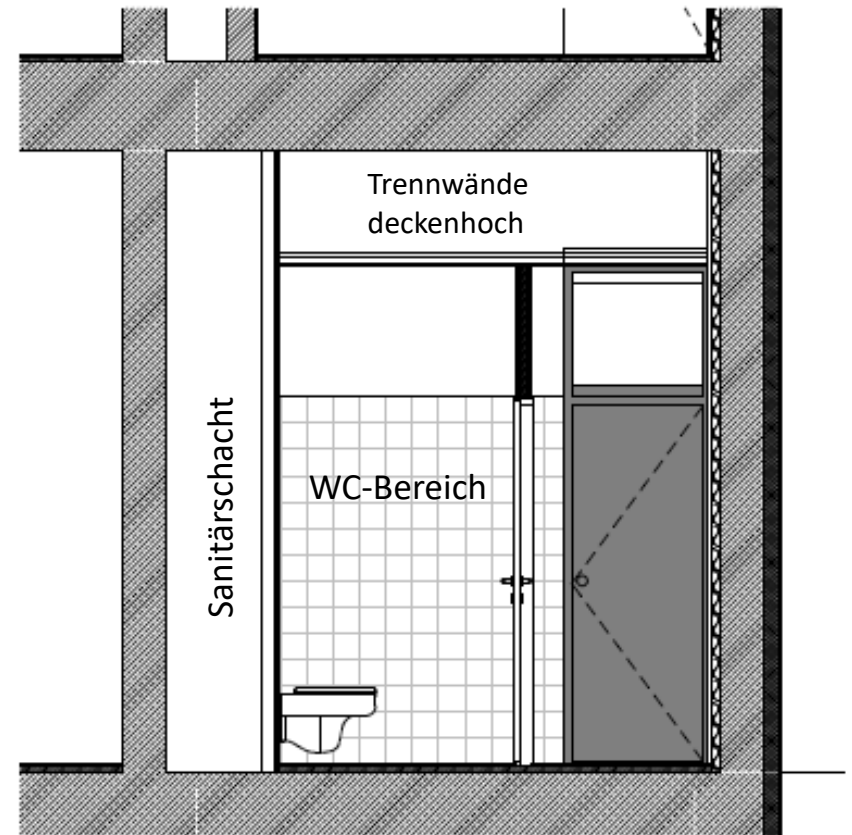
Schnitt WC-Bereich
