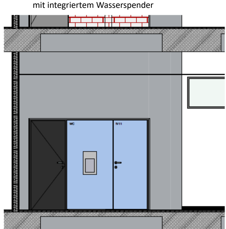
Schnitt/ Ansicht Zugang Flur
