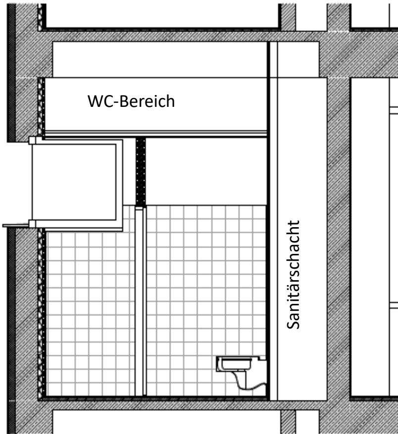
Schnitt WC-Bereich
