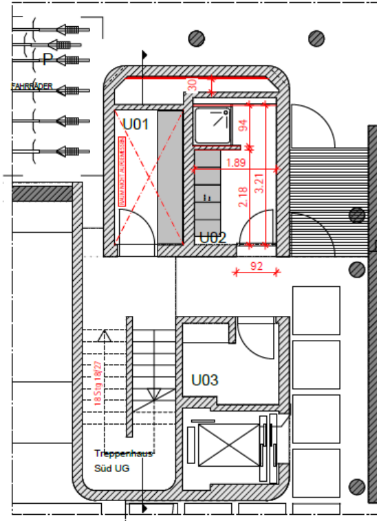
UNTERGESCHOSS BESTAND
