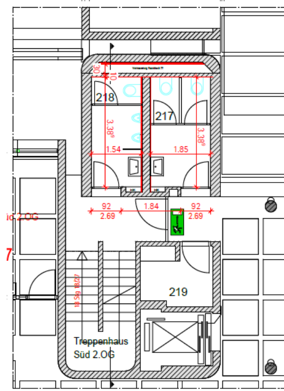
OBERGESCHOSS 2 BESTAND
