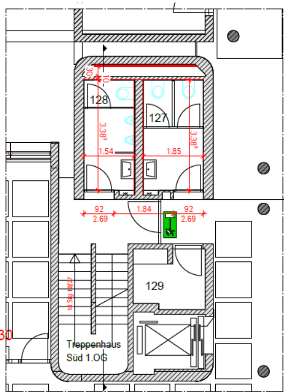
OBERGESCHOSS 1 BESTAND
