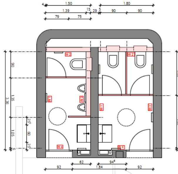
Grundriss
