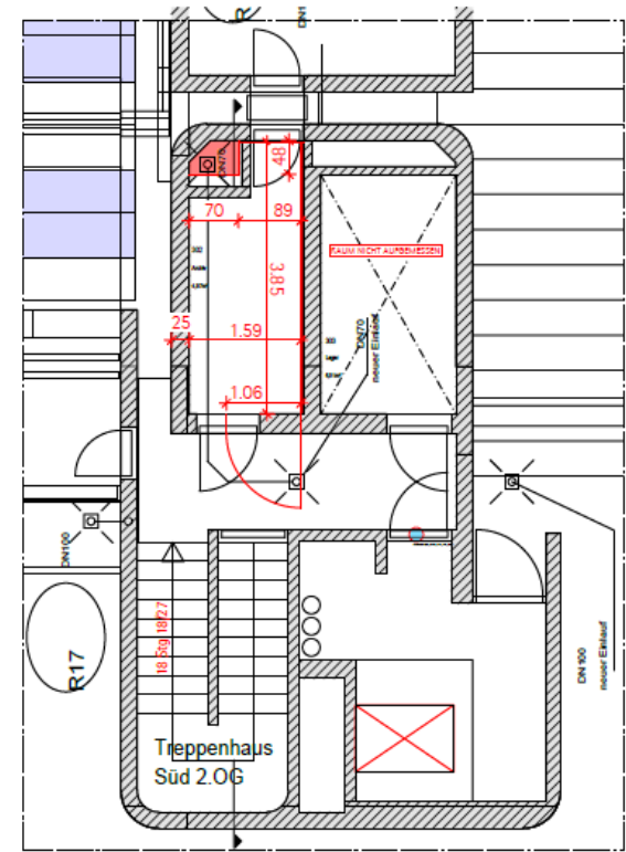
DACHGESCHOSS BESTAND
