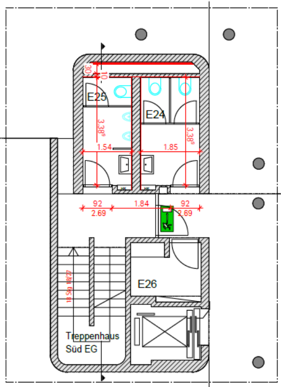
ERDGESCHOSS BESTAND
