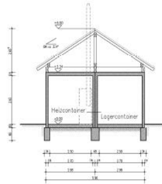
Schnitt A-A
